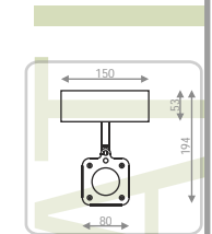
PHIL53 SO TOMA mini - CDM-Rm 35W anod.* 62500120 silver* 62500122 - halogen 12V 50W anod.* 62860120 silver* 62860122
