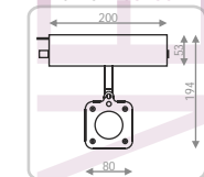
PHIL53 SK TOMA mini - CDM-Rm 35W (200mm) anod* 63240120 silver* 63240122 - halogen12V 50W (200mm) anod* 63250120 silver* 63250122
