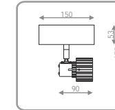
PHIL53 SO MAXI STAR TECHNO - halogen 230V 50W anod.* 62200120 silver* 62200122 - halogen 12V 50W anod.* 62220120 silver* 62220122 - CDM-Rm 35W anod.* 62240120 silver* 62240122
