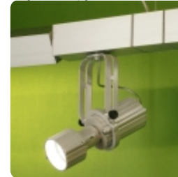
PHIL53 SO RETAKA - halogen 12V 50W anod.* 62100120 silver* 62100122 - CDM-Rm 35W anod.* 62110120 silver* 62110122
