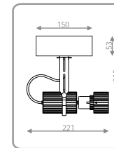
PHIL53 SO RETAKA - halogen12V 50W anod.* 62100120 silver* 62100122 - CDM-Rm 35W anod.* 62110120 silver* 62110122
