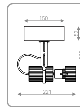
PHIL53 SO RETAKA - halogen 12V 50W anod.* 62100120 silver* 62100122 - CDM-Rm 35W anod.* 62110120 silver* 62110122
