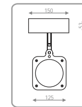
PHIL53 SO TOMA - CDM-R111 35W anod.* 62400120 silver* 62400122 - QR111 100W anod.* 62870120 silver* 62870122
