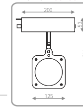
PHIL53 SK TOMA - CDM-R111 35W (200mm) anod* 63220120 silver* 63220122 - QR111 100W (200mm) anod* 63230120 silver* 63230122
