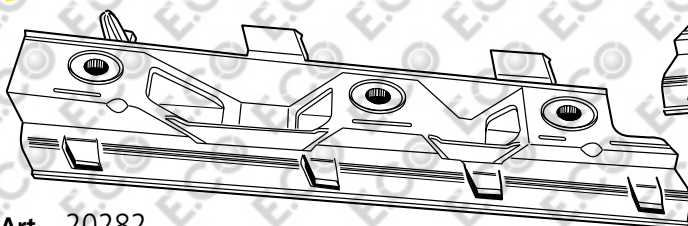
Art. 20282 Right bumper bracket Halter für Stoßstange rechts Скоба бампера, правая сторона OEM 3C0807184
