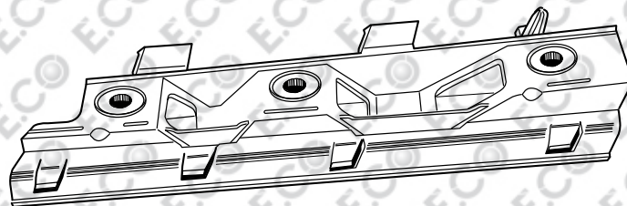
Art. 20283 Left bumper bracket Halter für Stoßstange links Скоба бампера, левая сторона OEM 3C0807183
