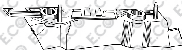
Art. 20277 Left bumper bracket Halter für Stoßstange links Скоба бампера, левая сторона OEM 8K0807283
